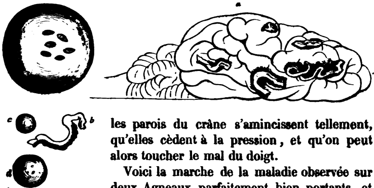
FIG. 174. — Tœnia cœnuro (*) (Cénure du Mouton).
